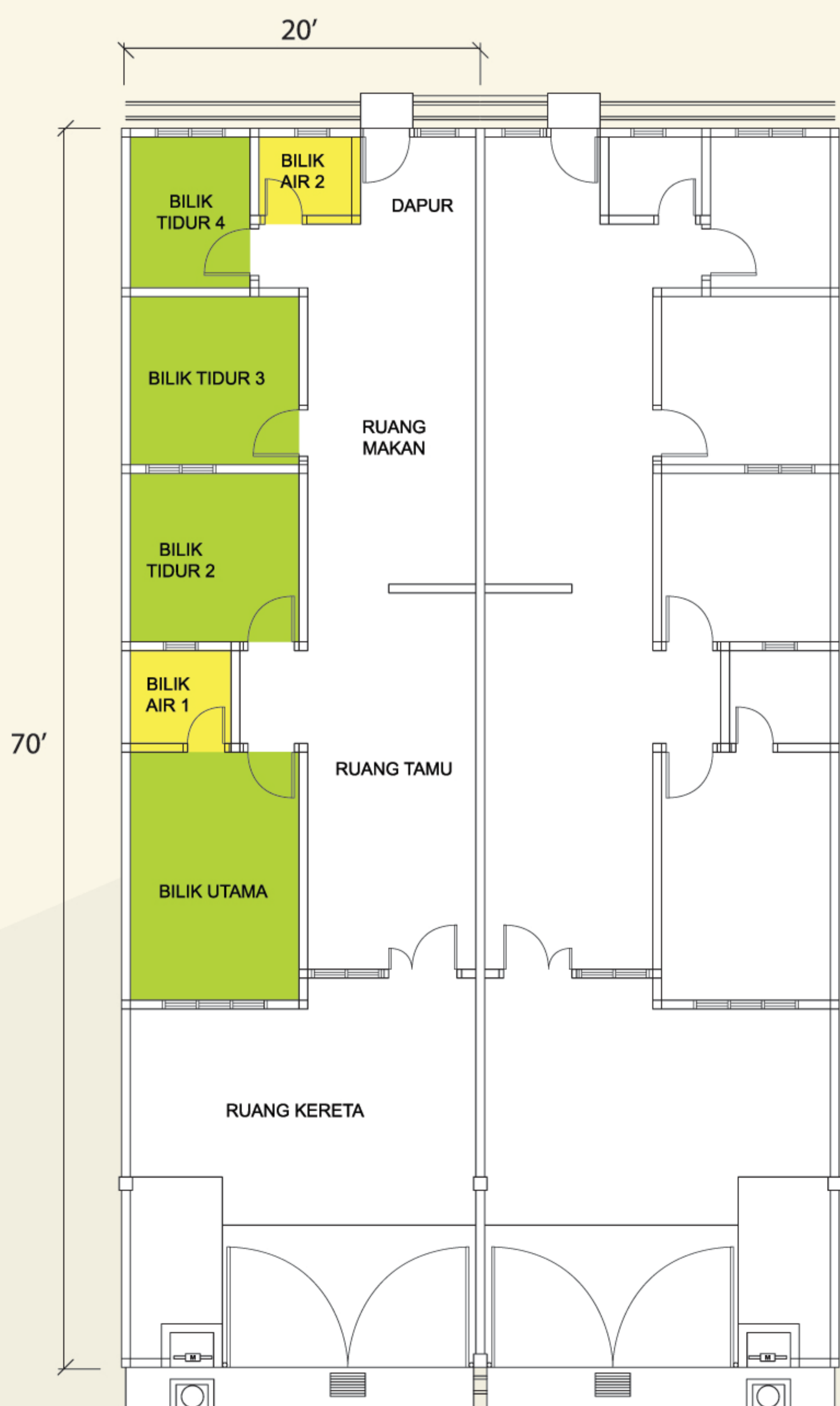
Pelan Lantai Luas Binaan: 1,264 kps
